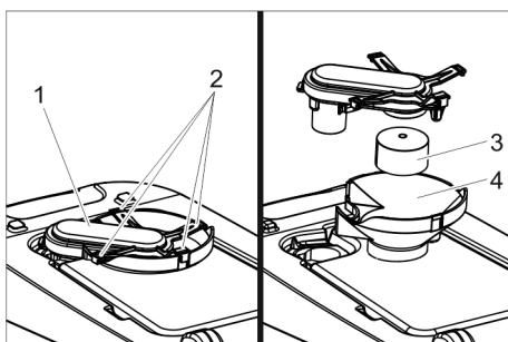
1 Boîtier flotteur
